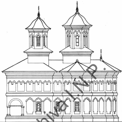
• VEDEREA LATERALA •
